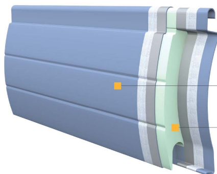
Lame aluminium profilé double paroi
